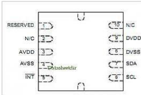
Fig 3: MEMS IC
