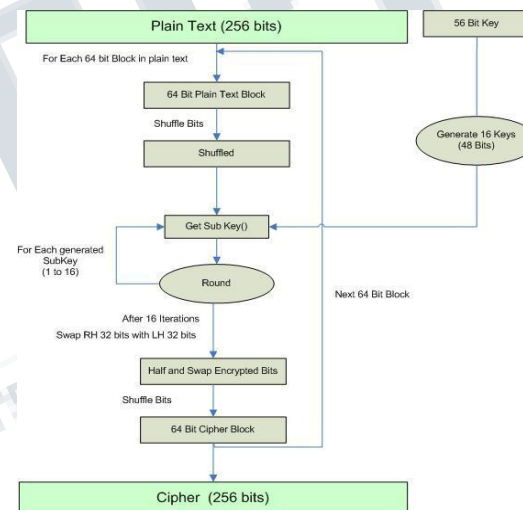
Fig-1. DES structure
